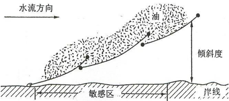
图 4-2 转移围栏
