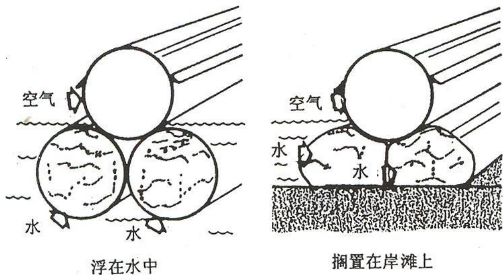
图 4-3 拦截围栏
