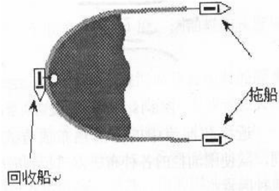
图 5-2 三船 U 型布放围油栏
